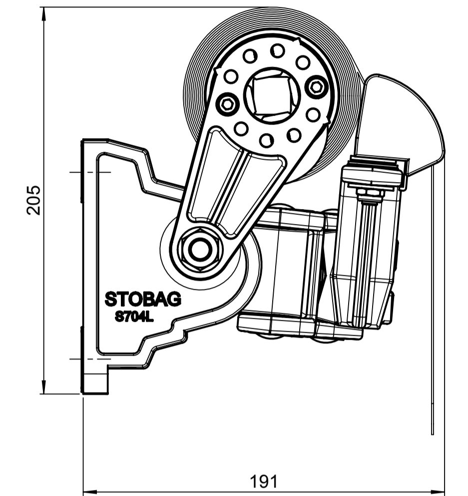
Wandmontage mit Motor
