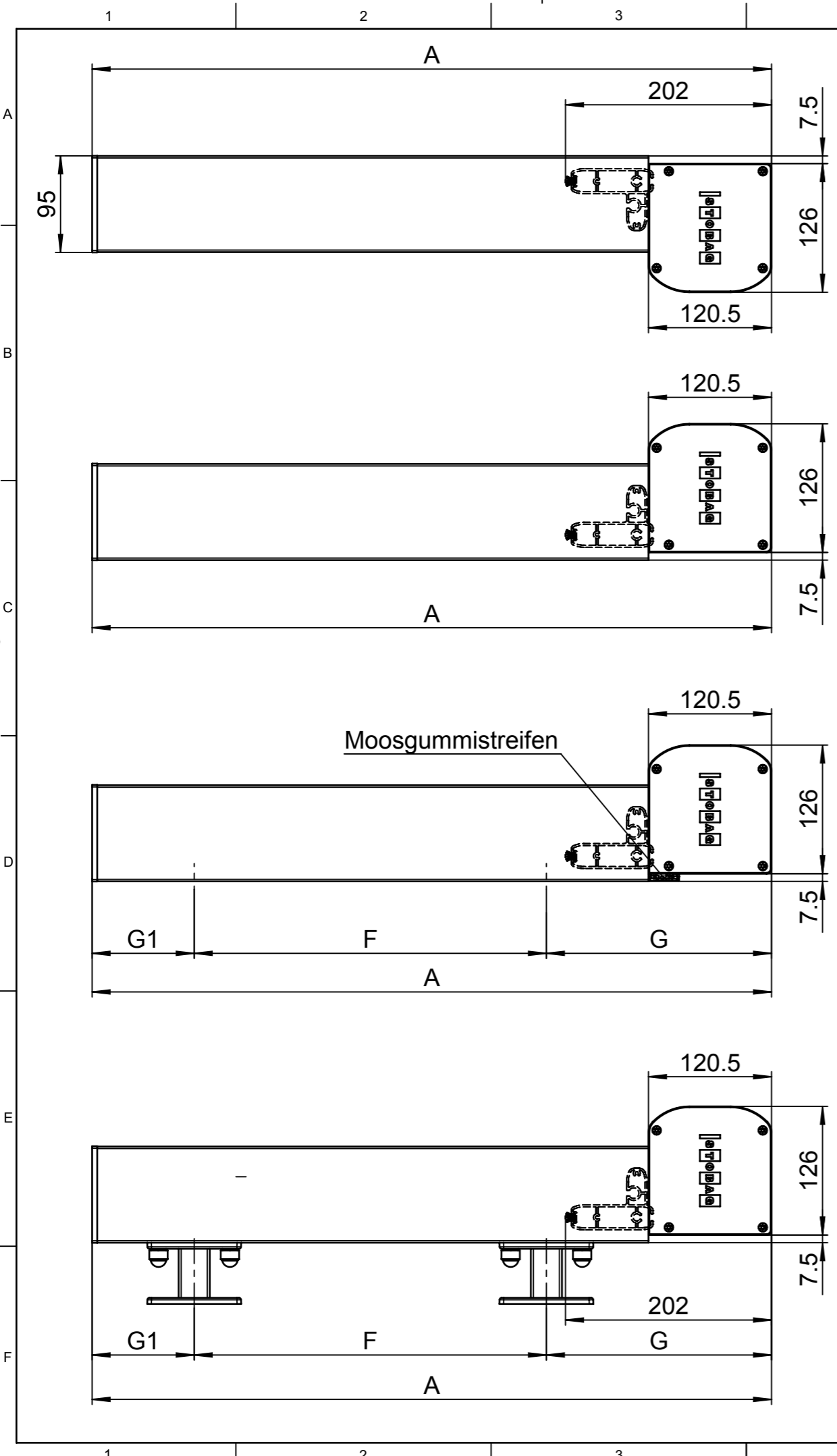
VD5400 Innenmontage
